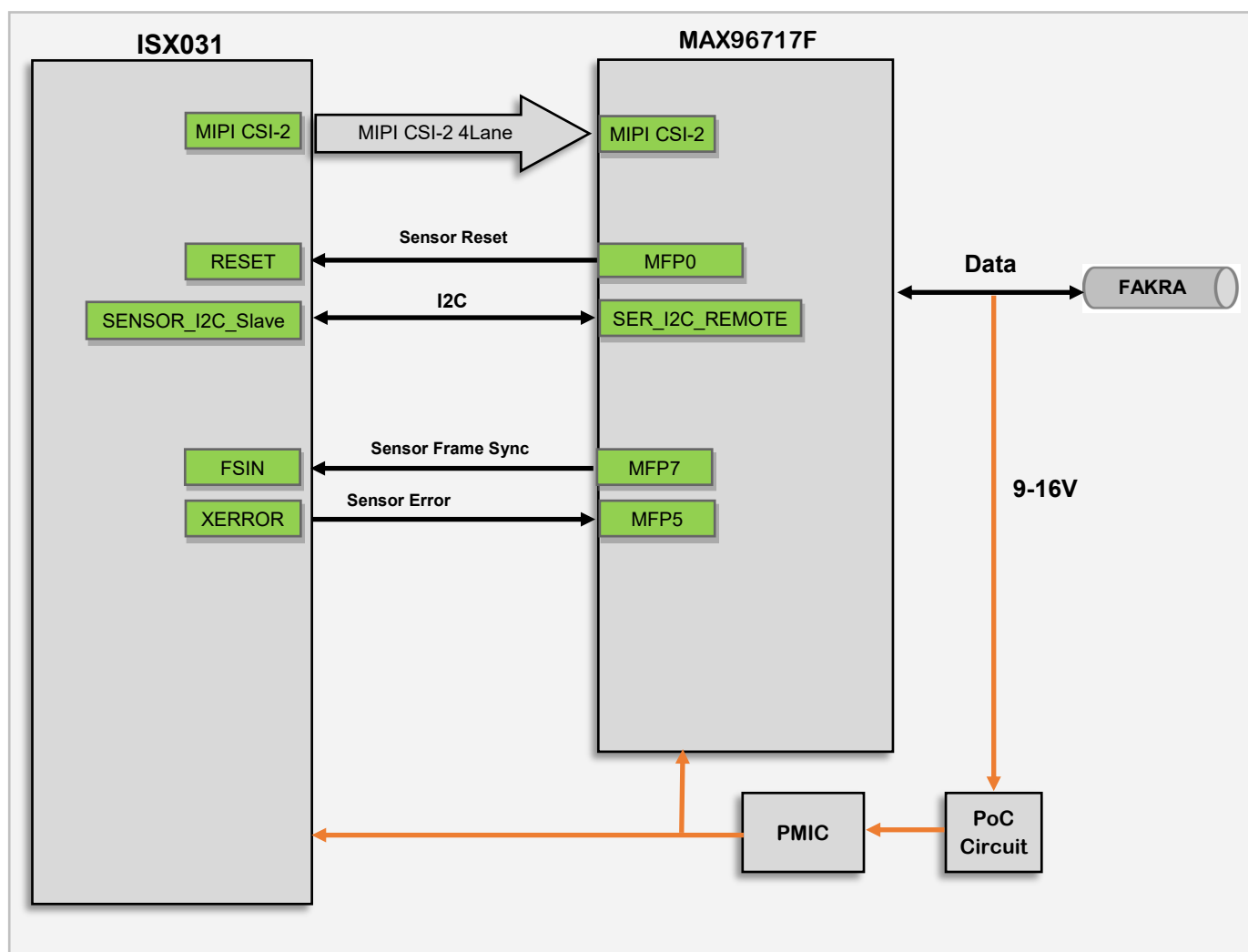
系统框图
